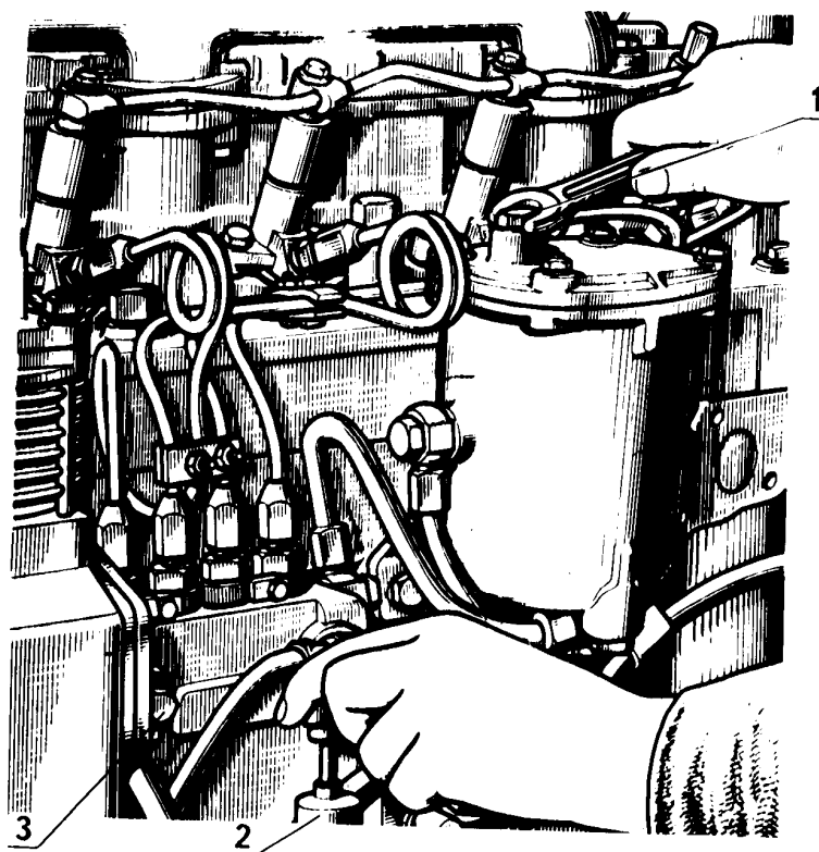
Рисунок 21 - Удаление воздуха из системы топливоподдачи.
