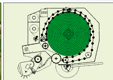
Прессовальная камера с цепным транспортером
